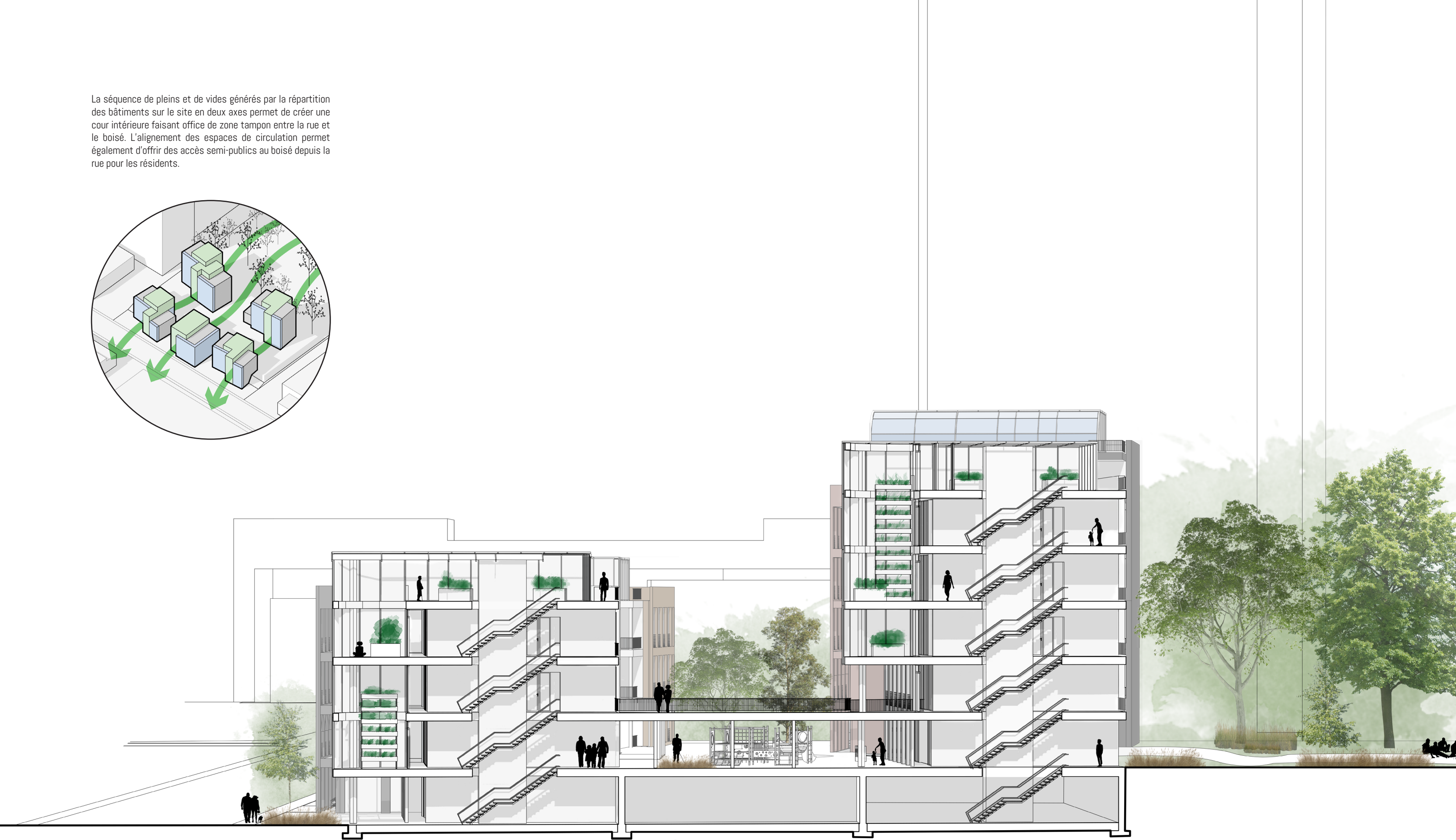
Coupe transversale
