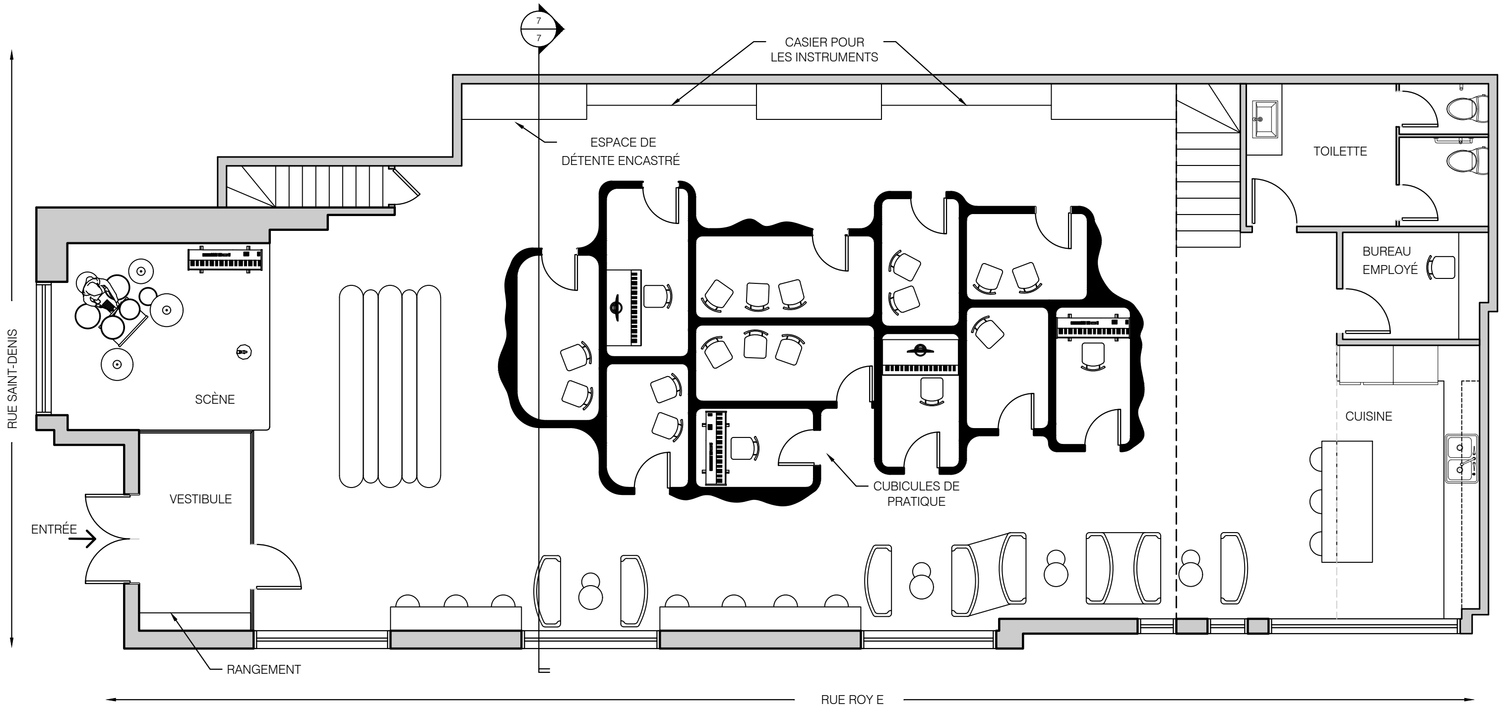
1 7 PLAN D'AMÉNAGEMENT ÉCH. : 3/16" = 1'-0"
