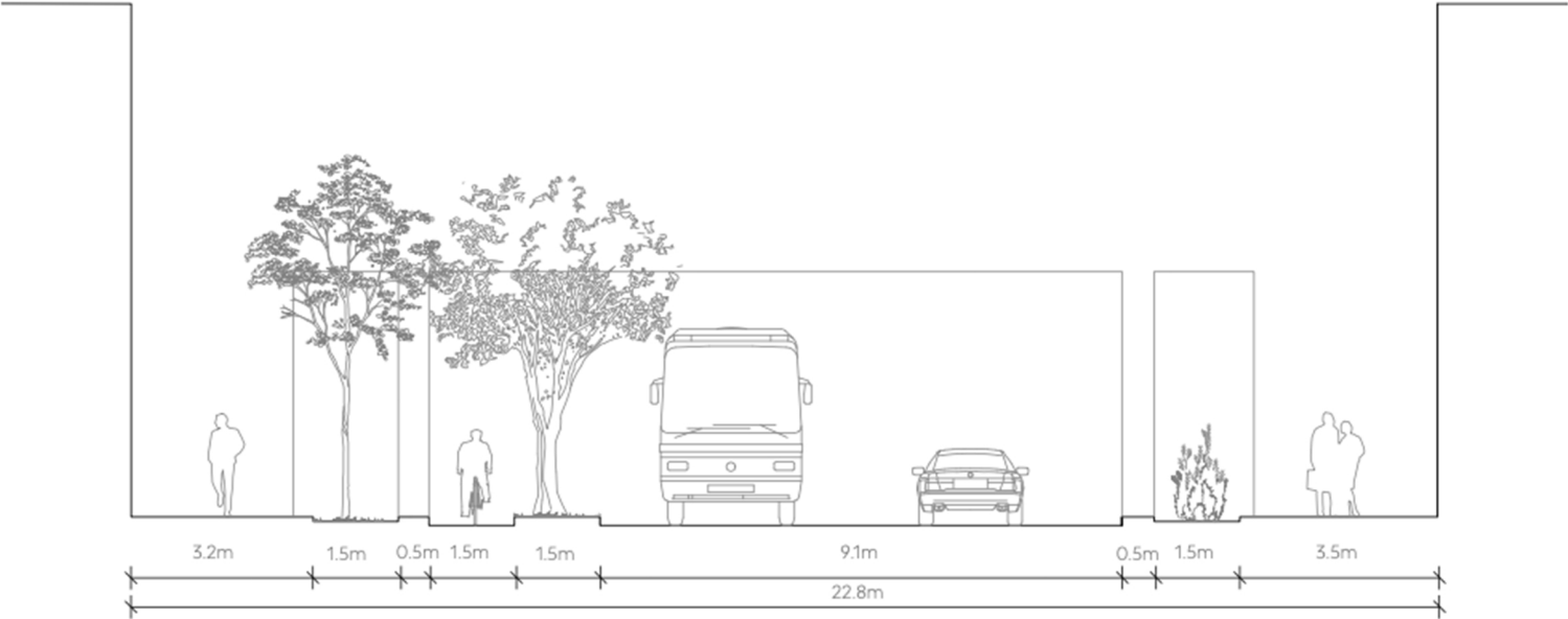
Coupe : rue Wellington. Échelle 1 : 100.
